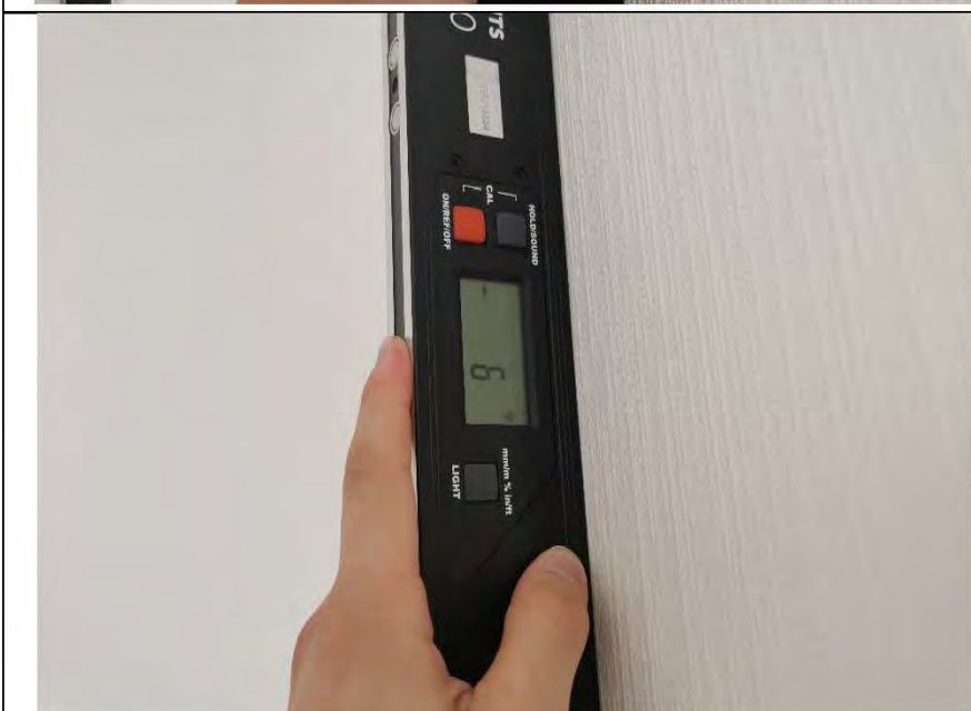
Фото №5. Измерение уровня стен в комнате.
