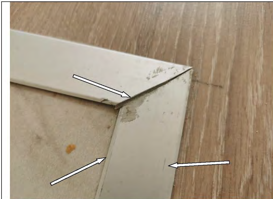
Фото №25. Механические повреждения напольного металлического плинтуса в кухне.
