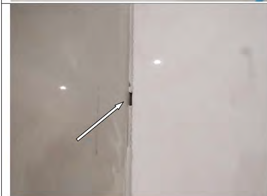
Фото №15. Неполное заполнение шовного пространства настенной керамической плитки затирачным составом в ванной комнате.
