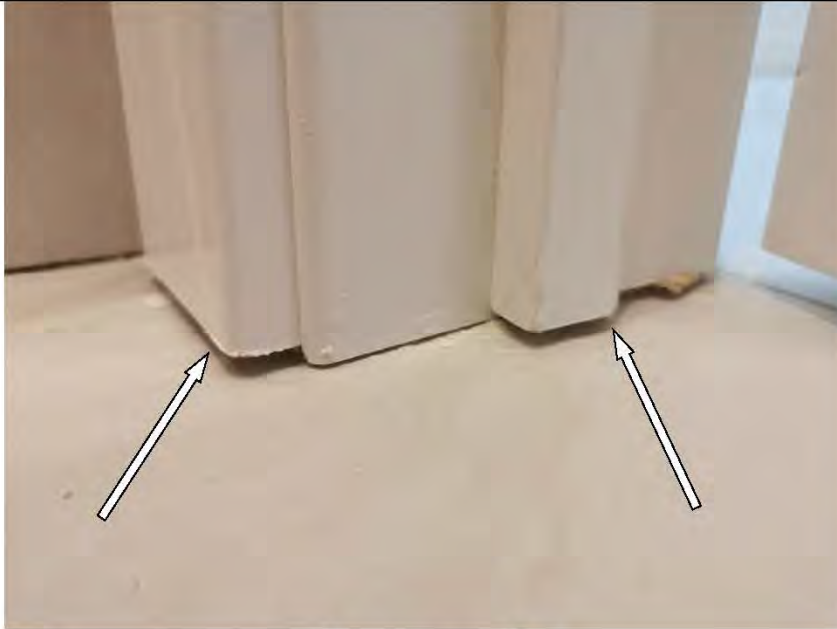
Фото №37. Коротко подрезаны коробка и наличник деревянного дверного блока в ванной комнате.
