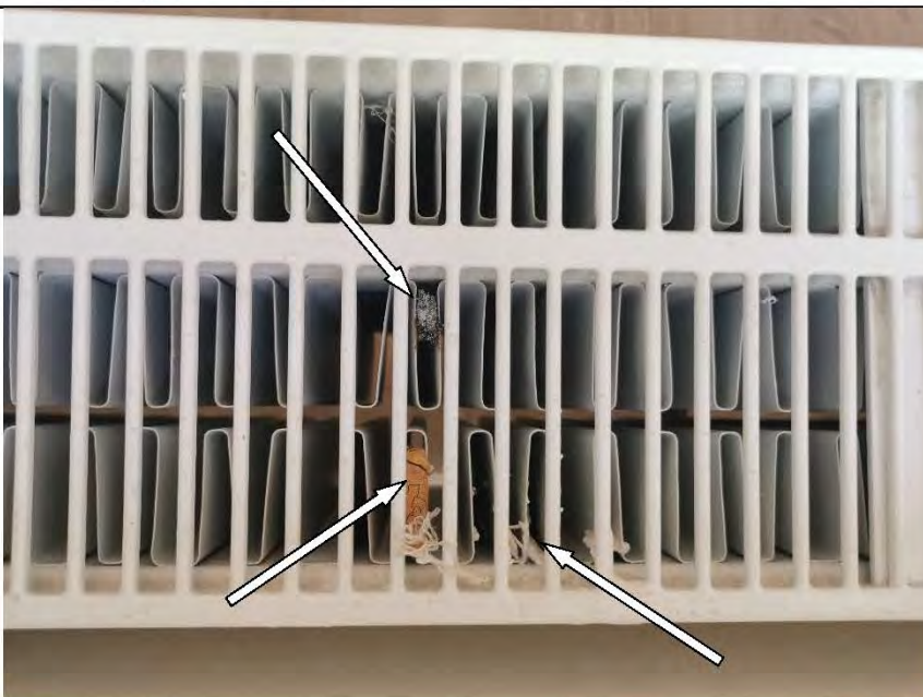
Фото №45. Загрязнение радиатора к комнате.
